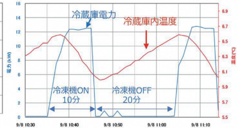
図2 冷蔵庫内の温度と消費電力推移
