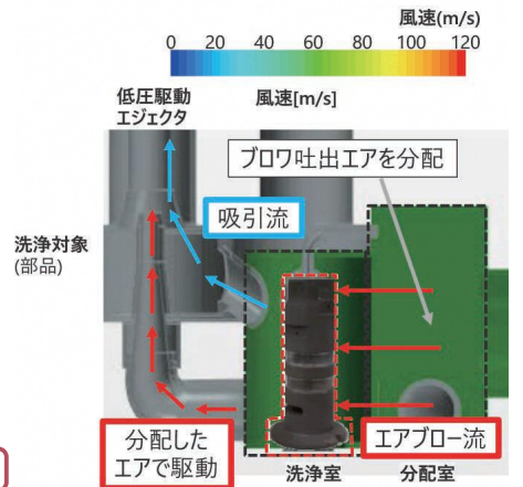
< 開発した一個洗浄システムの動作イメージ >
