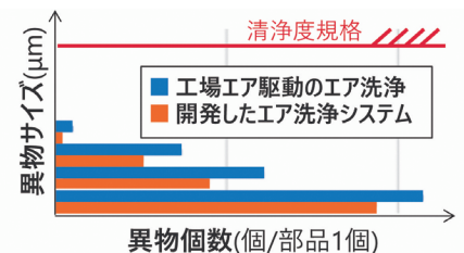
< 開発した一個洗浄システムの性能評価 >
