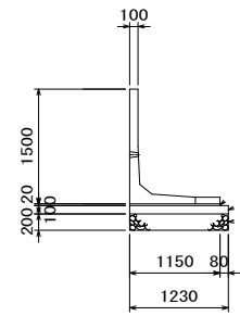
L型-1 (H1500)
