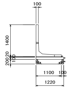
L型-1 (H1400)
