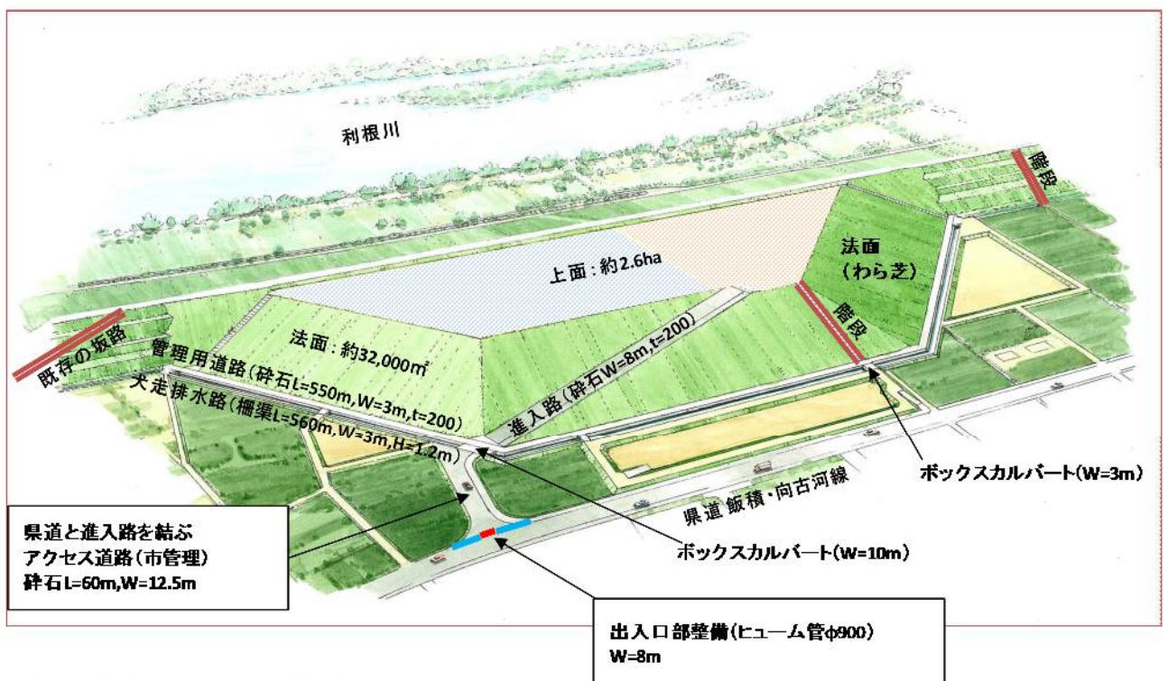
栄水防拠点整備イメージ図
