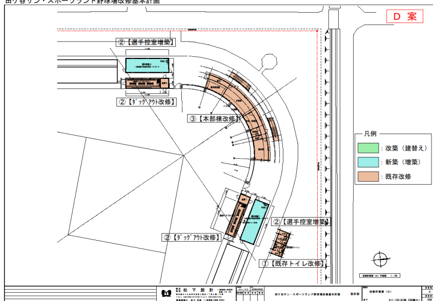
田ヶ谷サン・スポーツランド野球場改修基本計画
